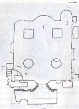
План храма Воскрешения Лазаря (придел церкви Рождества Богородицы) с аркосольной нишей в юго-западном углу — местом возможного погребения в 1399 г. княжны Марии, дочери Дмитрия Донского
