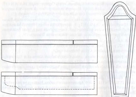
Саркофаг великой княгини Софьи, жены Василия I. 1453. План, разрезы
